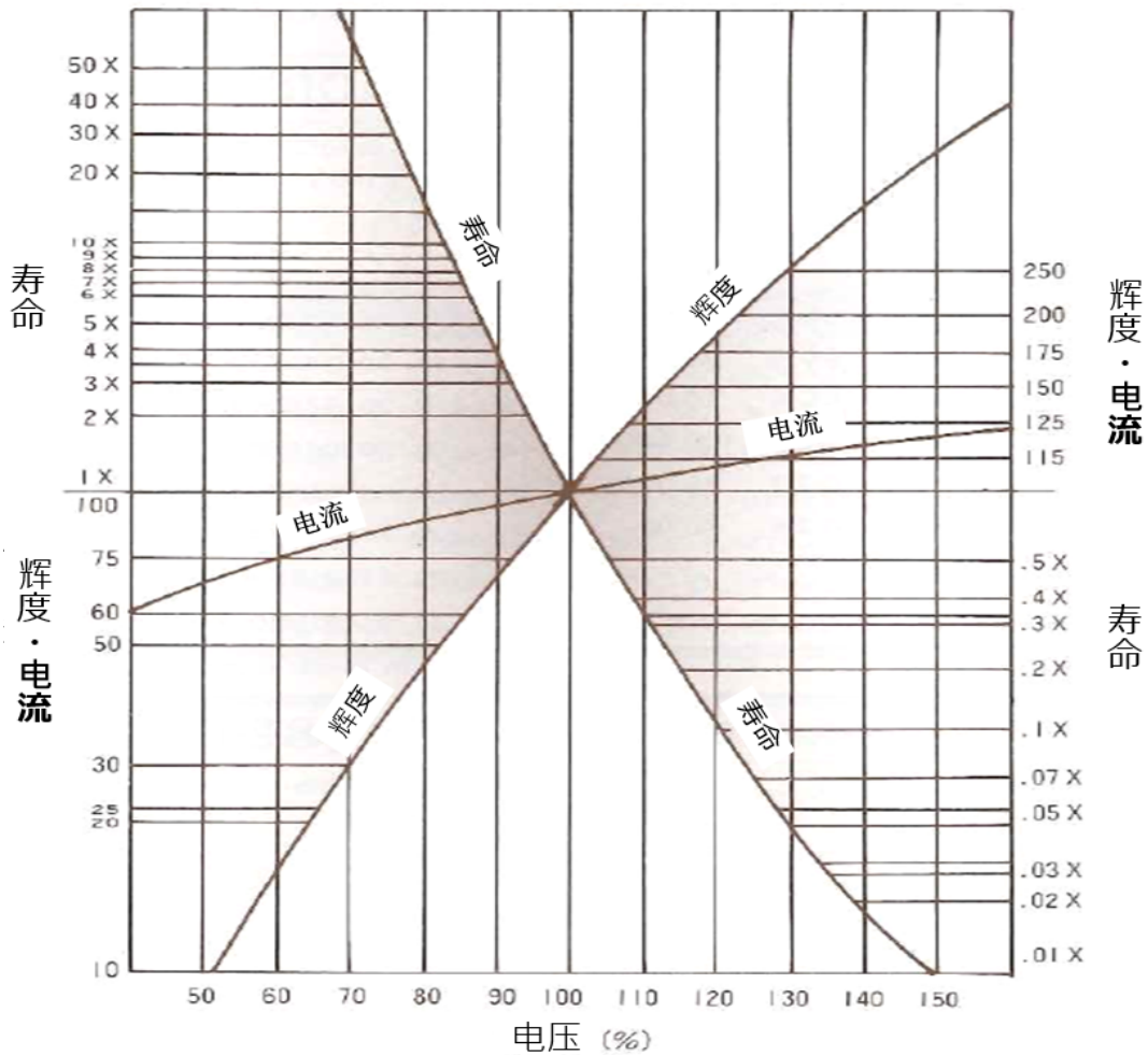
【过电压／低电压时的规格关联图】
